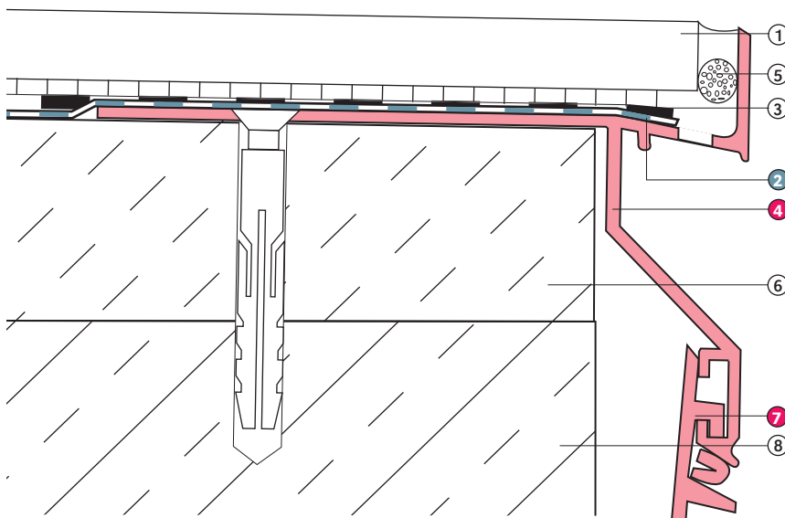
Detailabbildung 1:1
