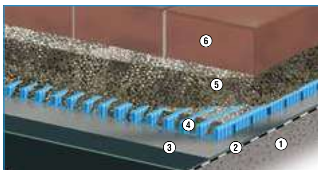
Revêtements de pavés roulable avec AquaDrain® HB
