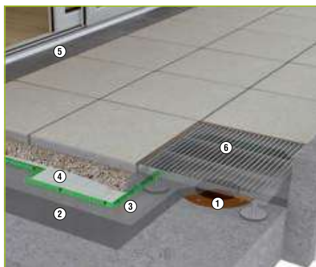
Grille d'écoulement AquaDrain® DR pour le drainage par le biais de siphons
