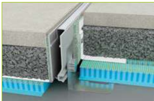
AquaDrain® SR-U pour l'évacuation linéaire
