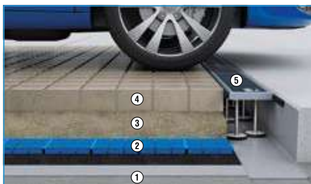
Drainage de type tunnel pour dalles de béton carrossables avec AquaDrain® HB-B pour optimiser l'évacuation de l'eau
