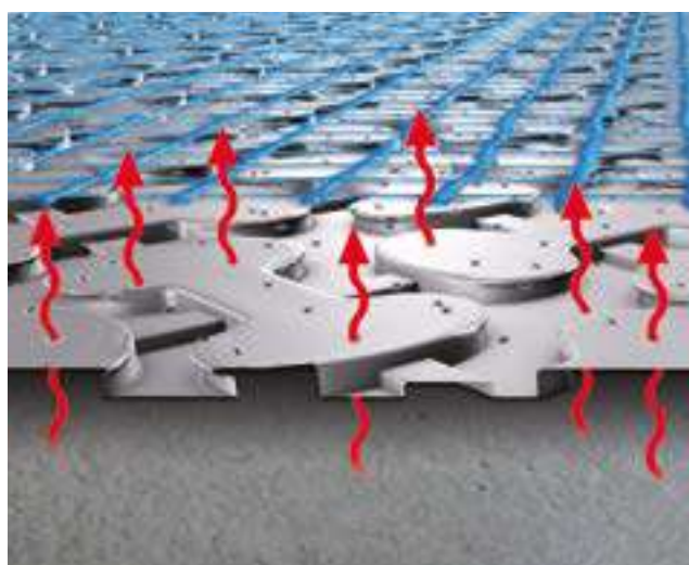
L'humidité restante dans le support se répartit de manière uniforme dans le système des canaux et peut s'évaporer au niveau des joints du revêtement grâce aux perforations de la natte.
