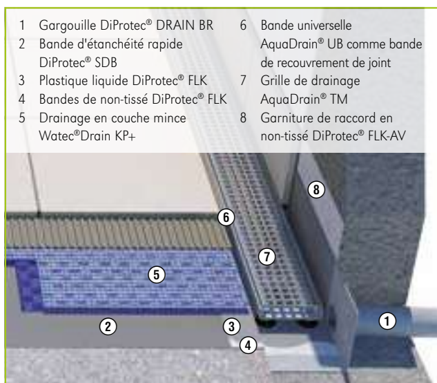
Balustrade de balcon avec évacuation linéaire des eaux et gargouille
