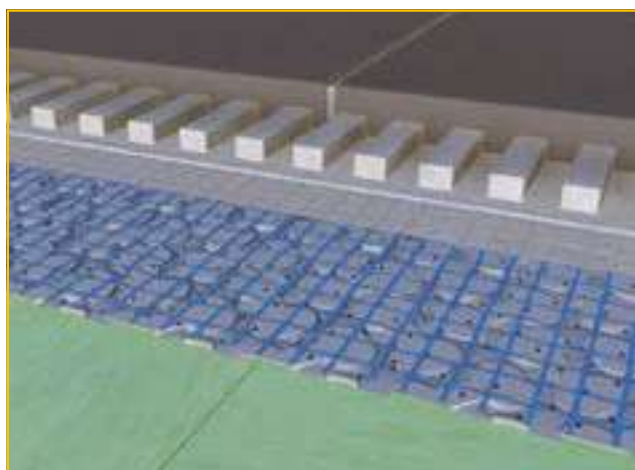
IndorTec® FLEXBONE-2E, la natte de désolidarisation en pose flottante pour les supports à mauvais accrochage (p. ex. le linoléum) avec un renforcement en treillis
