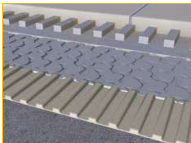
Désolidarisation des composites IndorTec® FLEXBONE-VA avec un non-tissé contrecollé sur la face inférieure
