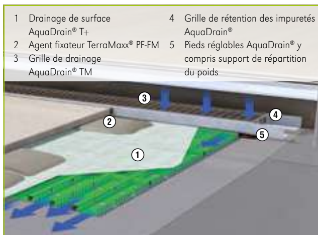
Pose en couche extrêmement mince TerraMaxx ® PF
