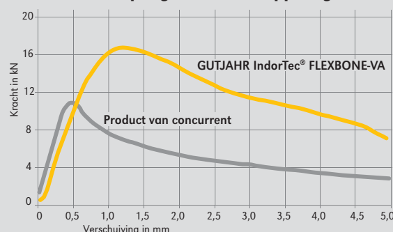
Afschuiftest op tegels met ontkoppelingsmat
