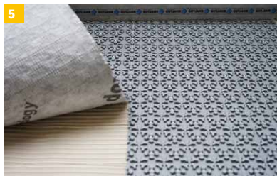
5 IndorTec® THERM-E in zugeschnittener Form mit dem Vlies in den Klebstoff einbetten.
